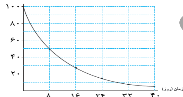
تعداد هسته‌های {}^{131}\text{I}
