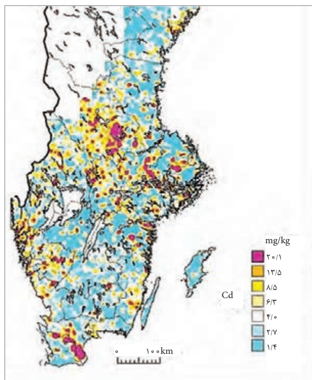
شکل ۳-۵- نقشه ژئوشیمیایی فلز سمی کادمیم در کشور سوئد
