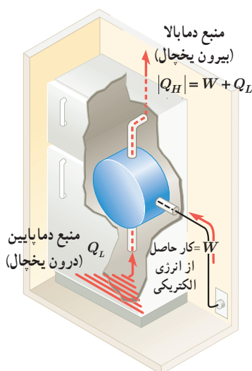
شکل ۸-۲۲ طرحی از طرز کار یک یخچال خانگی
