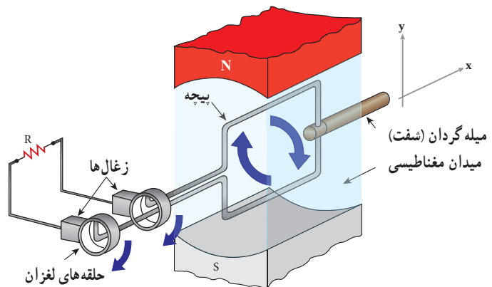
شکل ۳-۴ ا) اجزای یک مولد (ژنراتور) جریان متناوب. حرکت مکانیکی از طریق میله گردان، سبب چرخیدن پیچه در میدان مغناطیسی می‌شود و جریان متناوبی را در مدار به وجود می‌آورد.
