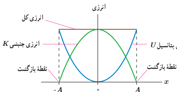
شکل ۳-۷ تبدیل انرژی در حین حرکت هماهنگ ساده سامانه جرم-فنر. توجه کنید که در نقطه x = 0 انرژی، صرفاً جنبشی و در نقطه‌های x = \pm A انرژی، صرفاً پتانسیل است. در این حرکت انرژی مکانیکی پایسته است، به گونه‌ای که به‌طور پیوسته از انرژی پتانسیل U به انرژی جنبشی K تبدیل می‌شود و بالعکس.
